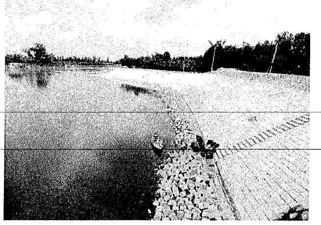
চিত্র: নদীতীর প্রতিরক্ষামূলক কাজ (ইছাপুর, পল্লীতলা, নওগাঁ, প্যাকেজ নং-Nao-W-4, টেন্ডার আইডি-৫১৮৬৯৮)
