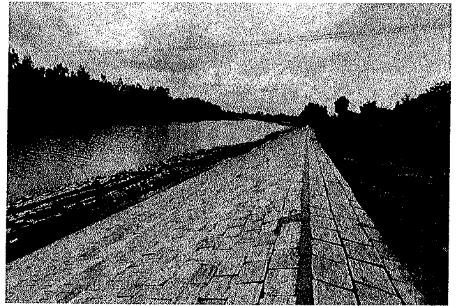
চিত্র: নদীতীর প্রতিরক্ষামূলক কাজ (কলোনীপাড়া, মহাদেবপুর, নওগাঁ, প্যাকেজ নং-Nao-W-3, টেন্ডার আইডি-৫১৮৬৯৭)
