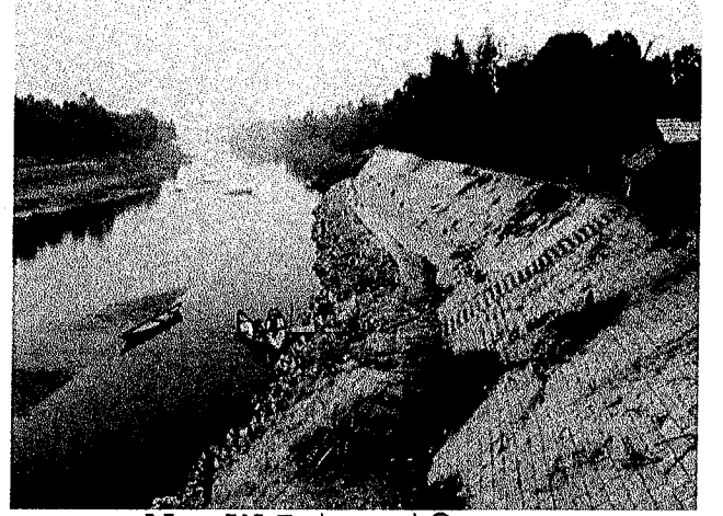
চিত্র: নদীতীর প্রতিরক্ষামূলক কাজ (উদয়শ্রী, খামুইরহাট, নওগাঁ, প্যাকেজ নং-Nao-W-5, টেন্ডার আইডি-৫৫৬১৫৬)
