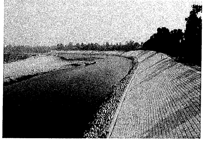
চিত্র: নদীতীর প্রতিরক্ষামূলক কাজ (পূর্ব পাটিচড়া, পল্লীতলা, নওগাঁ, প্যাকেজ নং-Nao-W-2, টেন্ডার আইডি-৫১৮৬৯৫)
